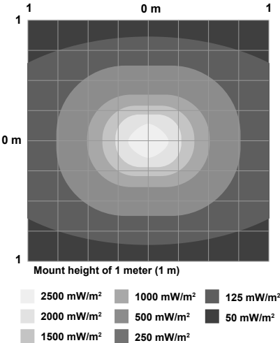
Iso-irradiance Pattern
