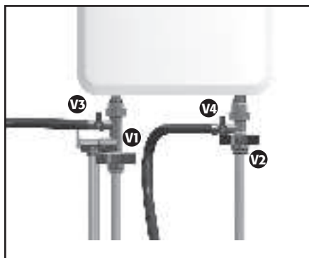
Figura 1 – Lavado del calentador de agua
