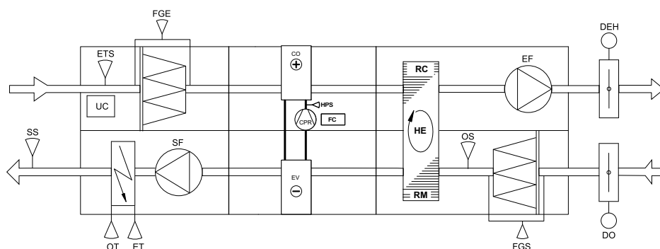
Рис. 4 Блок левого исполнения.
