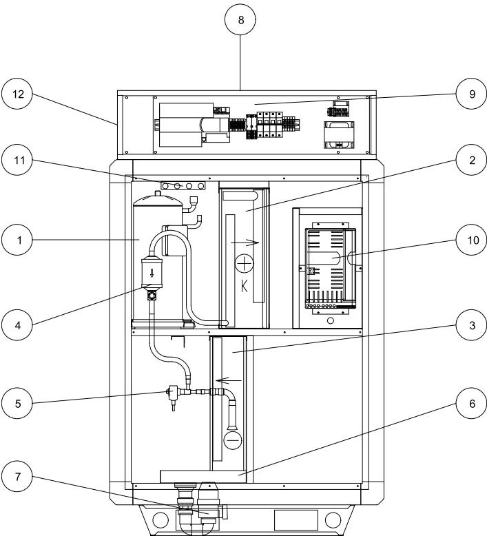
Рис. 1 Основные компоненты левостороннего агрегата
