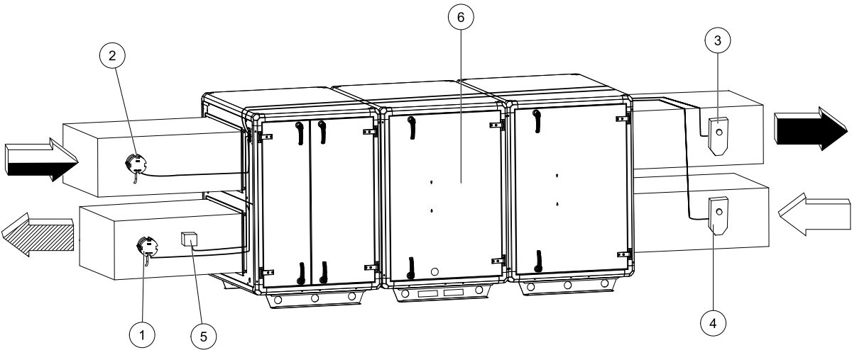
Рис. 3 Монтаж, левосторонний агрегат
