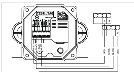
连接Axonic与CF800
