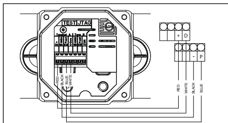
Collegamento AXONIC/CF800
