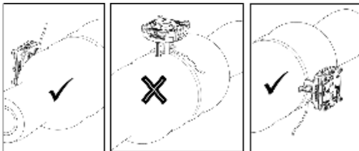
Abb.2: Ausrichtung des Zähler bei Medium-Temperatur 130...150°C
