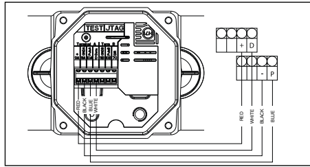
Anschluss Axonic an CF800
