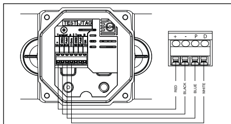
连接Axonic与CF51-CF55-PulseBox
