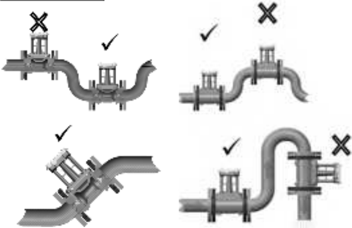
Fig N°3: Le mesureur doit toujours être rempli entièrement de liquide
