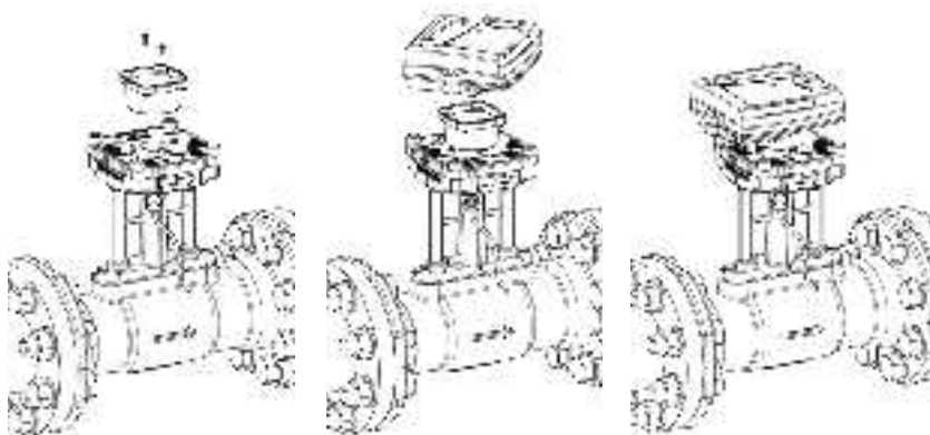
Abb.5: Befestigung Rechenwerk CF51 / CF55 direkt auf dem Axonic
