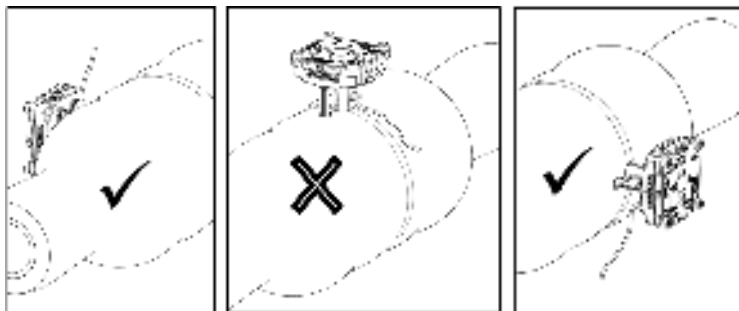
Рис. 2. Положение установки расходомер с теплоизоляцией при 130°- 150°С
