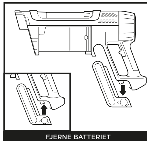
FJERNE BATTERIET
