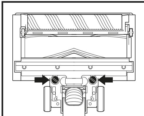
RIMOZIONE DEL TERGIPAVIMENTO
