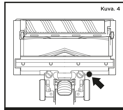
FLOORDETECT- LATTIANTUNNISTUSANTURI
