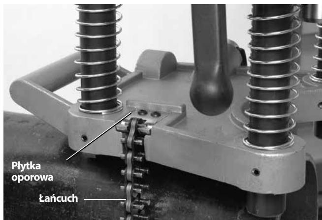
Rysunek 5 – Zahaczanie łańcucha w modelu HC-450
