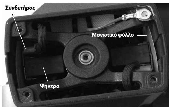
Εικόνα 12 – Τοποθέτηση ψήκτρας - Καπάκι μοτέρ έχει αφαιρεθεί
