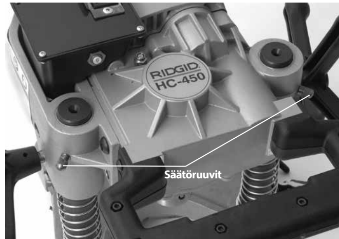
Kuva 13 – Säätöruuvien säätö
