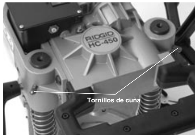
Figura 13 – Ajuste de los tornillos de cuña
