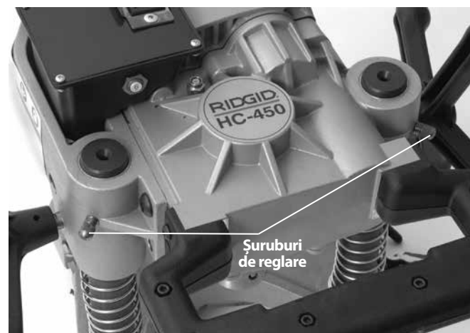
Figura 13 – Potrivirea șuruburilor de reglare
