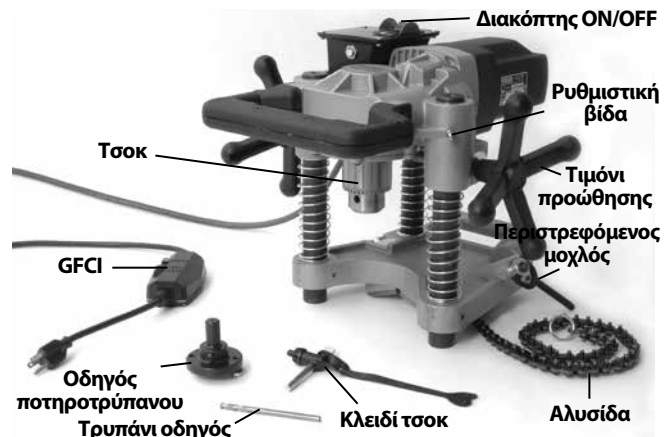
Εικόνα 1 – HC-450 με βασικό εξοπλισμό
