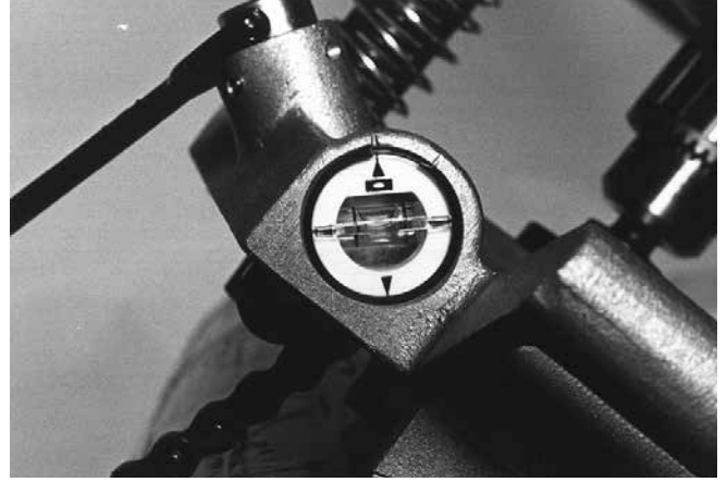
Şekil 6 – HC-450 Delik Açma Makinesi Düzleme Terazisi Göstergesi
