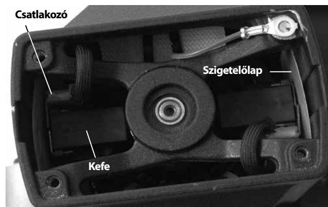
12. ábra – A kefe elhelyezése - motorburkolat eltávolítva
