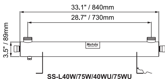
SS-L40W/75W/40WU/75WU
