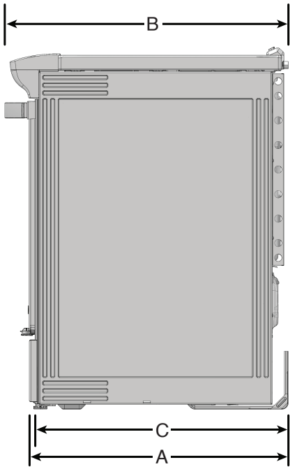
VISTA LATERAL
