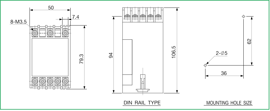
EVR-PD
