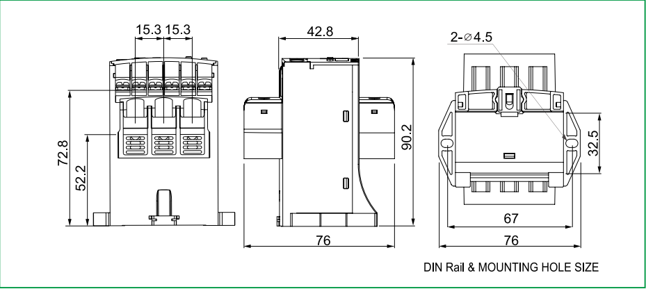
EOCR-DS1T / DS3T
