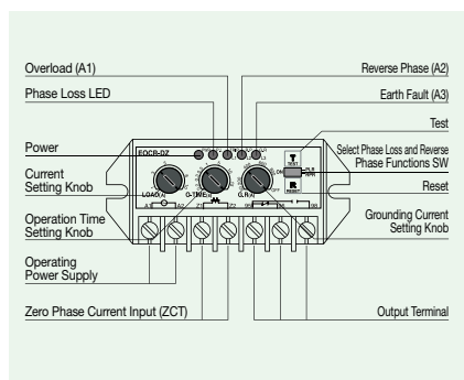
EOCR-DZ
