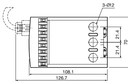
PANEL & DIN RAIL TYPE
