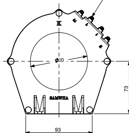
ZCT-Ø80
