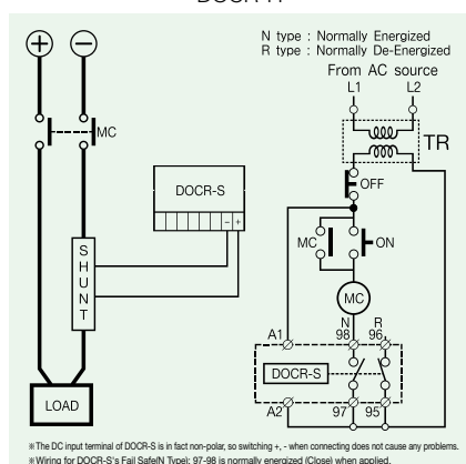
DOCR-H
