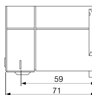
DIN RAIL TYPE
