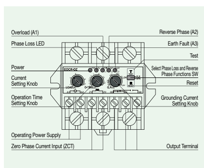
EOCR-DZT
