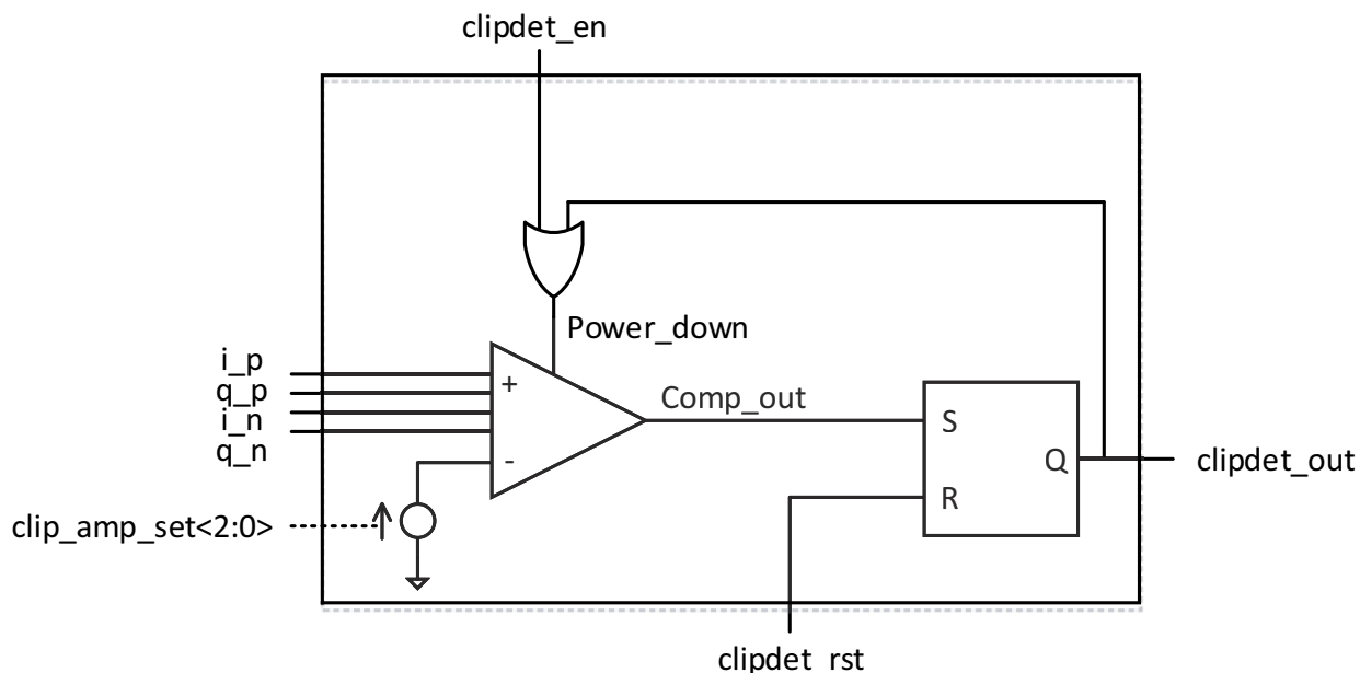
Fig 117. Clip detector 2
