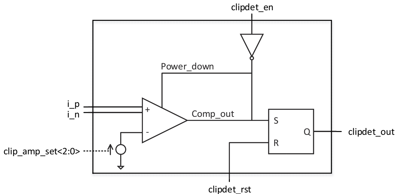
Fig 116. Clip detector 1
