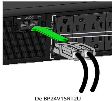
Figure 1. Conexión de BP24V15RT2U al UPS
