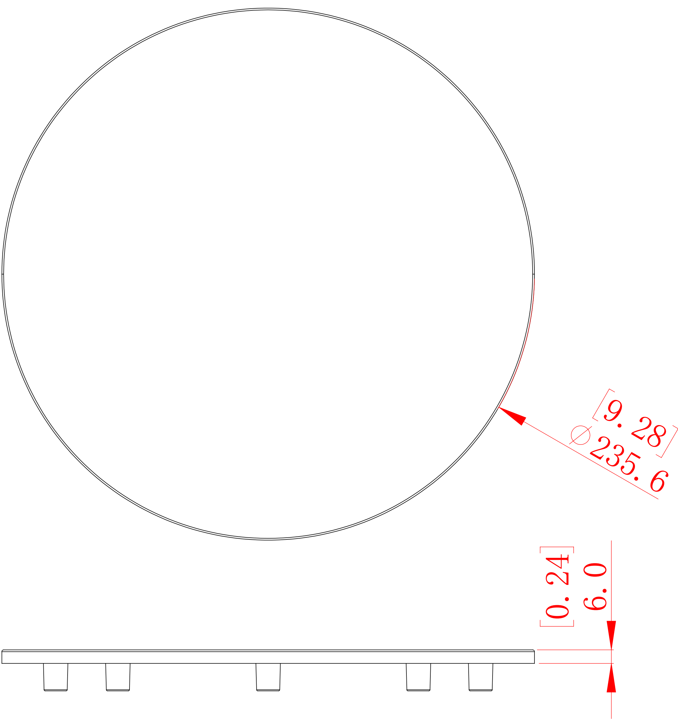
TRIMLESS GRILLE
