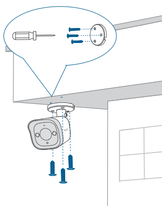
På taket
