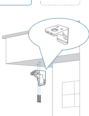
Takmontering
