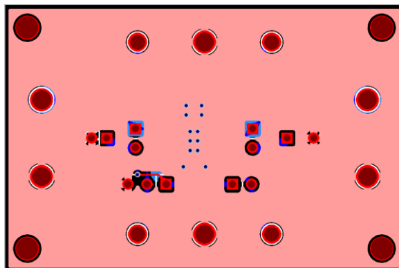
Figure 31. AP21X1AS-EVM – Bottom Layer
