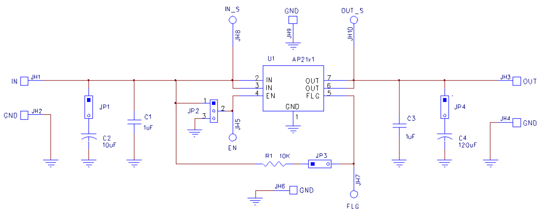
Figure 15. AP21X1AS-EVM
