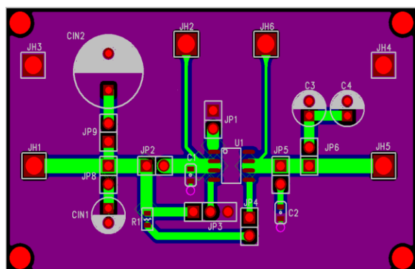
Figure 22. AP21X1AS-EVM – Top Layer
