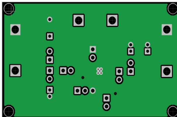
Figure 19. AP21X1AMP-EVM – Bottom Layer
