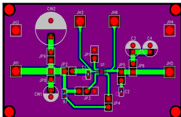
Figure 20. AP21X1AFM-EVM – Top Layer
