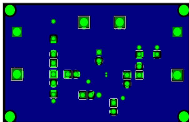
Figure 21. AP21X1AFM-EVM – Bottom Layer
