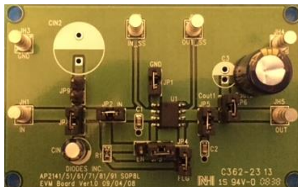
Figure 4. AP21X1AS-EVM
