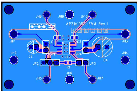
Figure 30. AP21X1AS-EVM – Top Layer
