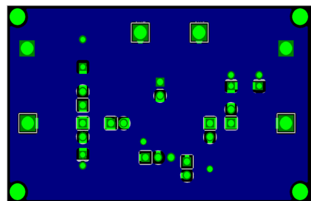
Figure 23. AP21X1AS-EVM – Bottom Layer
