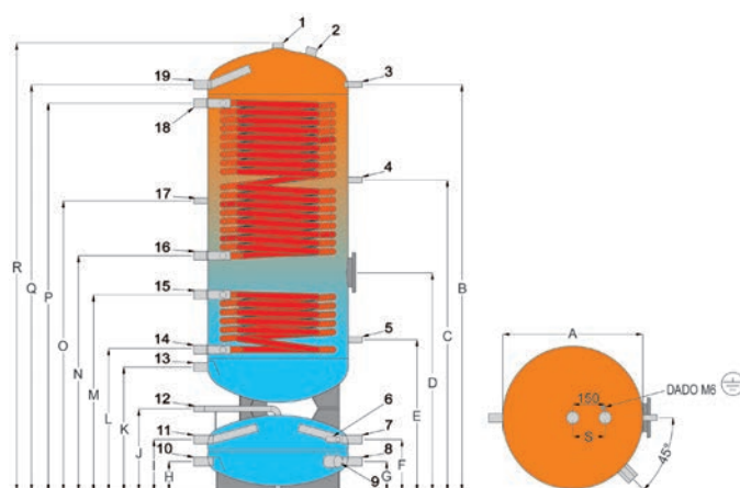
HYS Bollitore 2 serpentine (per PdC + solare + serbatoio inerziale)
