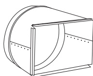
Transición del conducto cilíndrico de 8" x 12" a 12"
