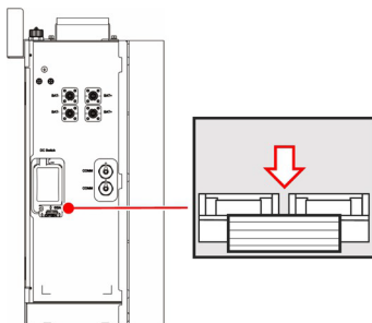
Slika 13: Isključivanje strujnog prekidača
