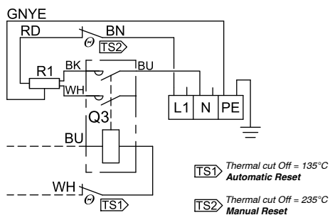
DETTAGLIO COLLEGAMENTO ELETTRICO ELECTRIC HEATER WIRING DETAIL SZCZEGÓŁ POŁĄCZENIA ELEKTRYCZNEGO
