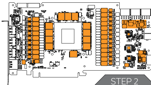
Thermal Pad F 1.0mm
