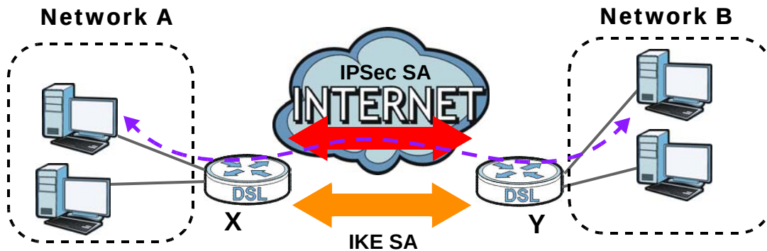
Figure 146 VPN: IKE SA and IPsec SA
