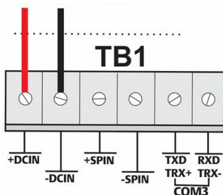
Abbildung 9. Verkabelung zur DC-Spannungsversorgung (ohne optionalen E/A)
