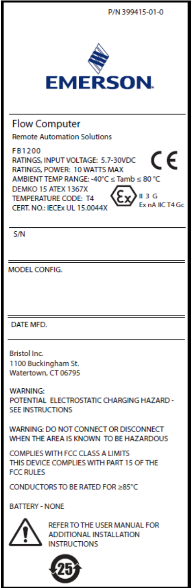
图2. 艾默生FB1200 标签（无火花）
