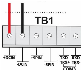
Afbeelding 9. Bedrading naar gelijkstroomvoeding (zonder optionele I/O)
