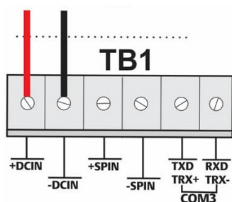
Figura 9. Fiação à fonte de alimentação CC (sem E/S opcional)
