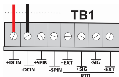
图8. 接线至直流电源（带可选I/O）
