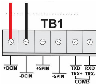
Figura 9. Cableado de la fuente de alimentación de CC (sin E/S opcional)
