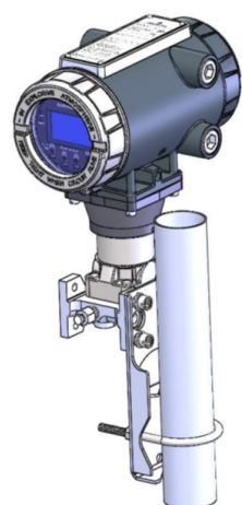
图7. 管道安装座上的FB1200
