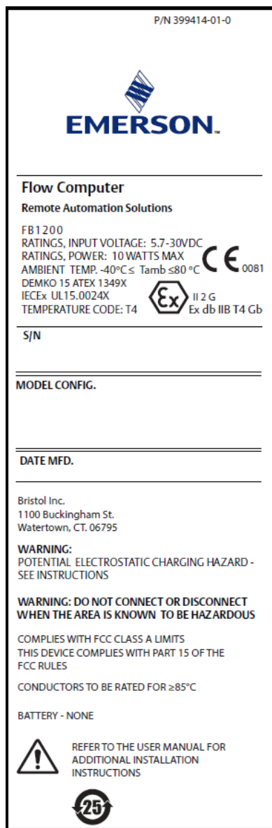
Figure 1. Étiquette Emerson FB1200 (antidéflagrant)
