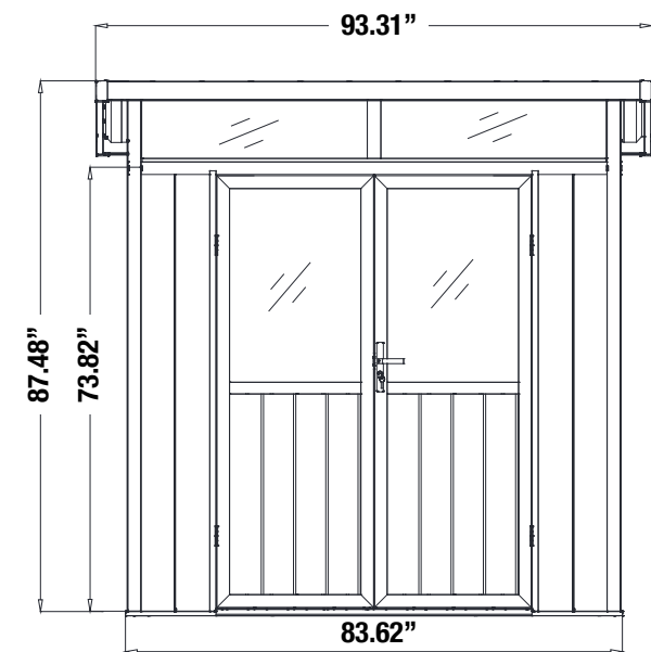
EN FRONT VIEW FR VUE FRONTALE
