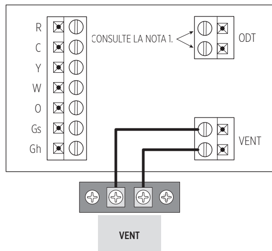
FIGURA 8: CABLEADO DEL MODELO 8120X
