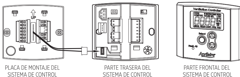
FIGURA 12: CONEXIÓN DEL SISTEMA DE CONTROL AL VENTILADOR
