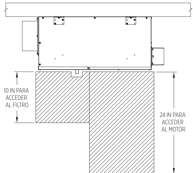
FIGURA 2: ESPACIOS PARA REALIZAR EL MANTENIMIENTO
