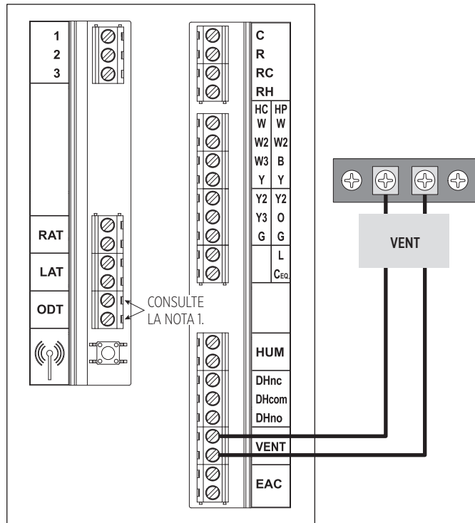
FIGURA 5: CABLEADO DEL SISTEMA DE CONTROL DE IAQ
