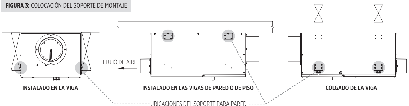
FIGURA 3: COLOCACIÓN DEL SOPORTE DE MONTAJE
