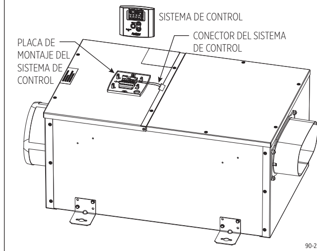
FIGURA 9: RETIRO DEL SISTEMA DE CONTROL DE LA PLACA DE MONTAJE
