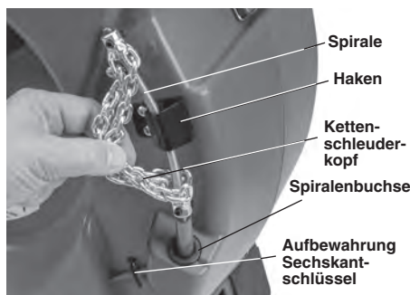
Abbildung 1C – Spiralenende/ Kettenschleuderkopf
