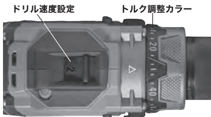
図6-ドリルの設定
