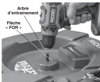
Figure 4 – Montage de la perceuse sur l'arbre d'entraînement
