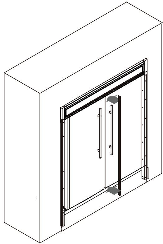
8 Fix the middle decorative partition Fixer la cloison décorative centrale
