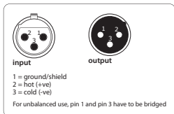
XLR-kontakt (stiften är utmärkta på kontakten)
