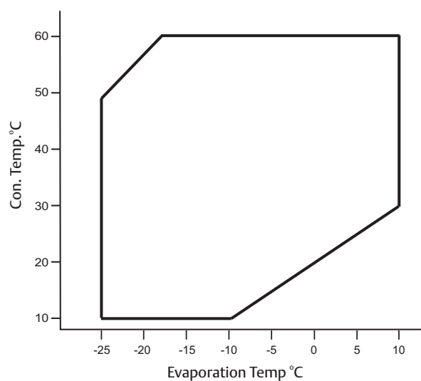
ZB15KQE~ZB76KQE, ZB92KCE~ZB11MCE R404A/507
