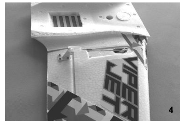
Bild 4 – Verbinden Sie die Anlenkstange mit dem Servo und den Ruderhorn.
