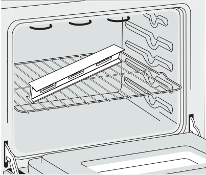
Figure 8: Nivelación
