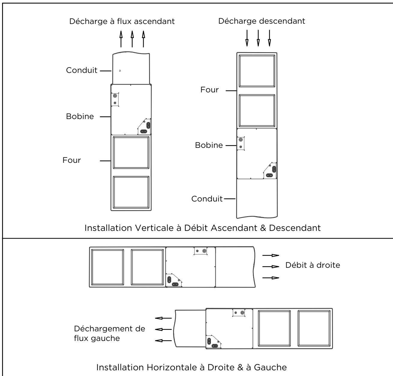
Type d'installation 2 : Modèle MMC60H2128B installation de la bobine sur le four
