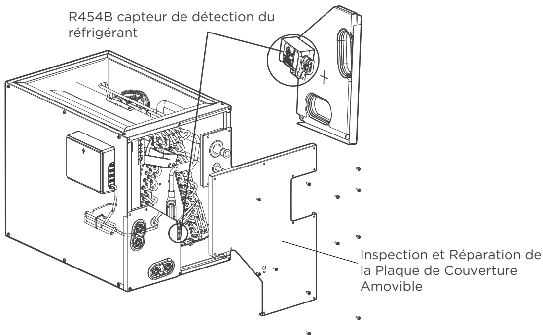
DIMENSIONS DU BOÎTIER ET EMPLACEMENT DES COMPOSANTS
