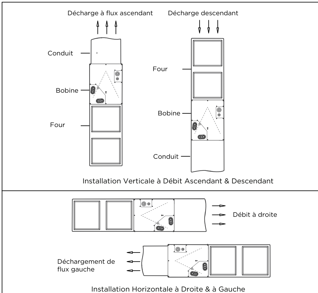
Type d'installation 1 : Installation typique d'une bobine sur un four
