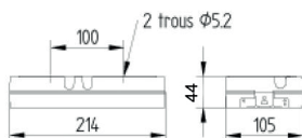
Ultraled 8 - Dimensions (mm) (produit monté avec fond ou patère existant)
