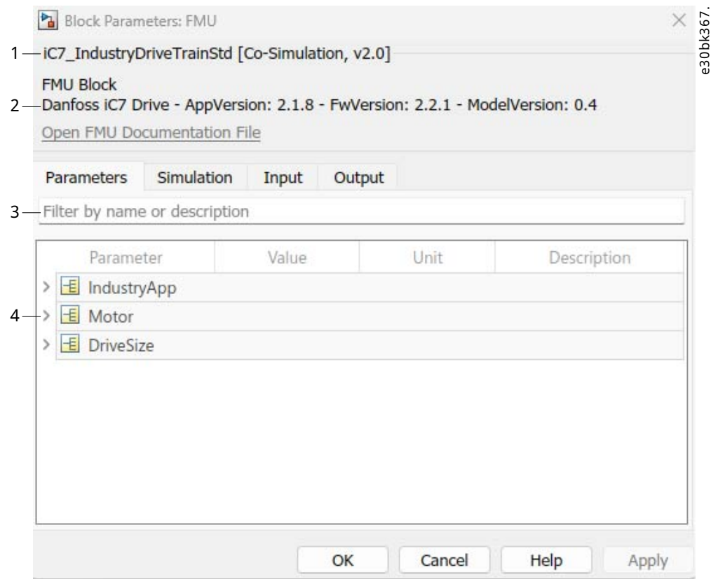
Figure 1: Parameter Menu in Simulink
