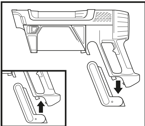
FJERNE BATTERIET
