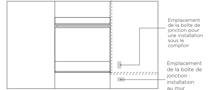
Emplacements des boîtes de jonction
