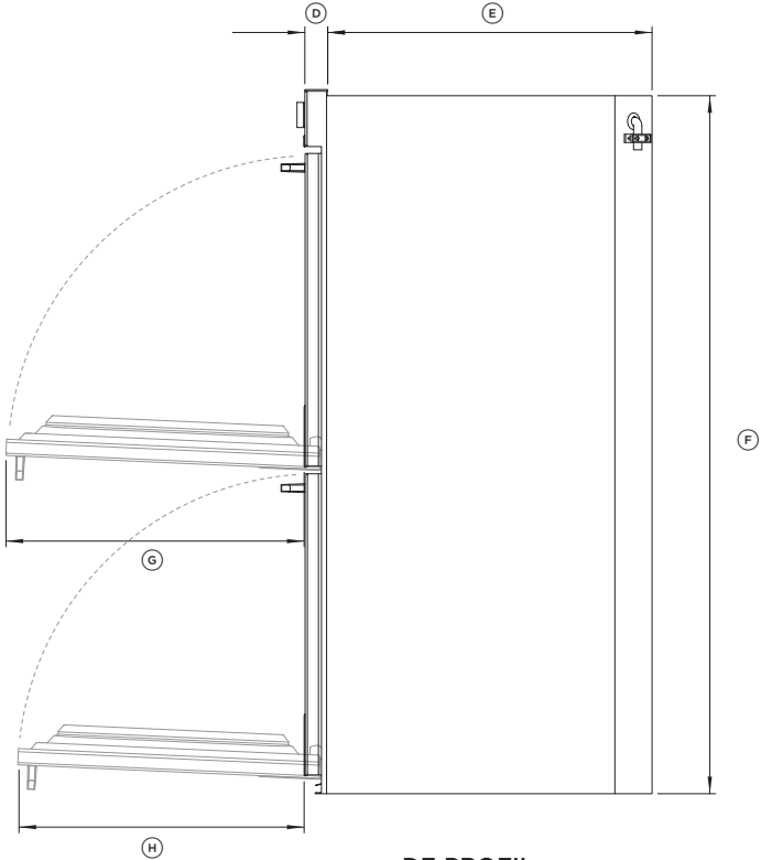
DE PROFIL
