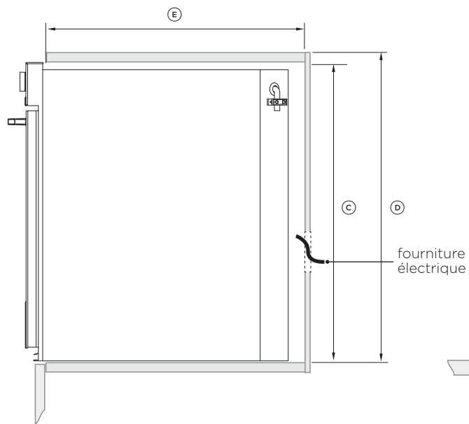
DE PROFIL
