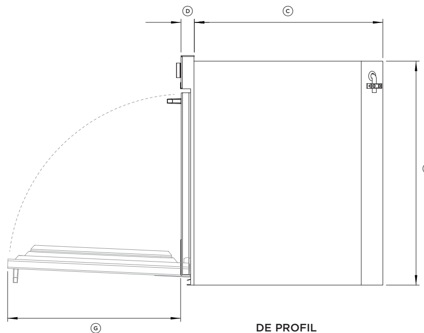
DE PROFIL
