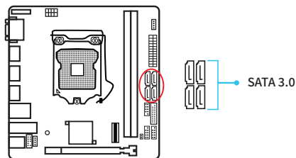
2-12 SATA接口
