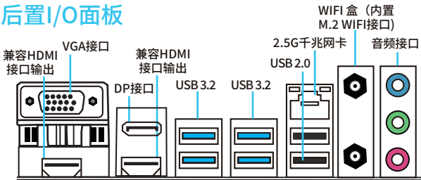
1-2 整体后置I/O面板展示
