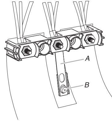
A. Barrette de liaison à la terre métallique
