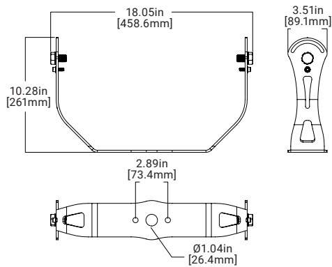
PENDANT MOUNT
