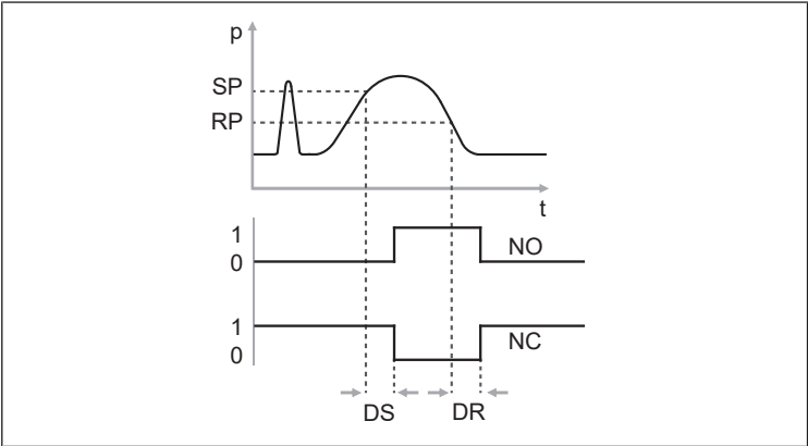
Abb. 6: Verzögerungszeiten
