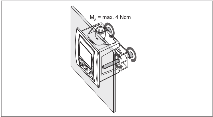
Abb. 16: Mit Befestigungsschrauben fixieren und kontern
