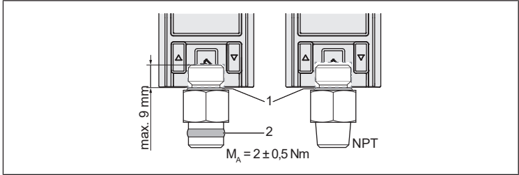
Abb. 17: Doppelnippel für Drucksensor (1 = O-Ring, 2 = Dichtungsring PTFE)
