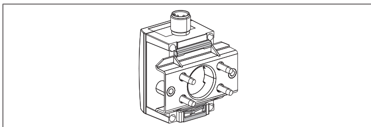
Рис. 11: Крепежный комплект с установленным на нем датчиком давления
