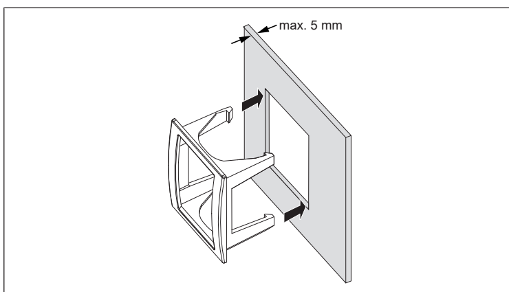
Рис. 13: Установить лицевую рамку в вырез
