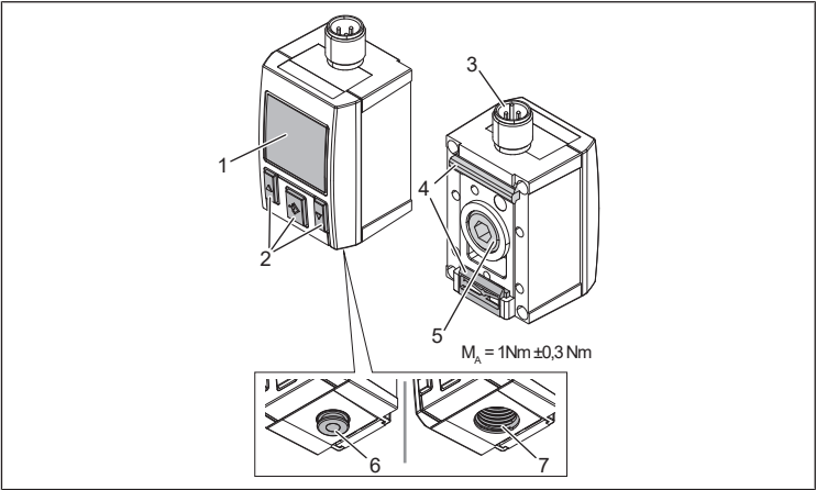
Abb. 1: Geräteübersicht
