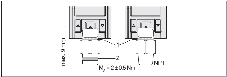
Fig. 17: Boquilla doble para sensor de medición de presión (1 = junta tórica, 2 = anillo obturador de PTFE)
