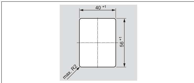
Рис. 12: Отверстие в панели
