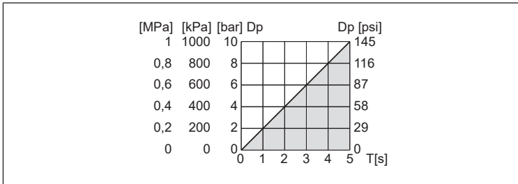
Fig. 18: Durée de période T admise (zone grise) en fonction de la variation de pression \Delta p
