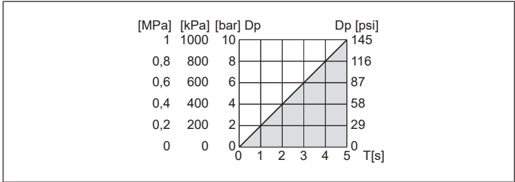
Fig. 18: Durata T consentita (area grigia) in funzione dell'oscillazione della pressione \Delta p
