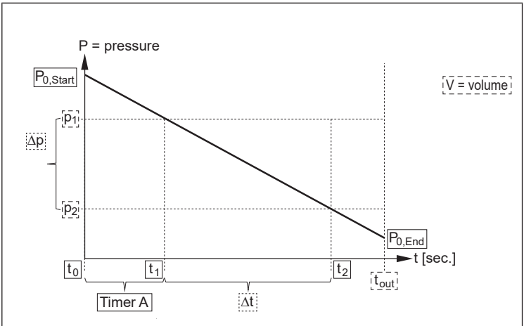
Abb. 23: Leckagekennlinie
