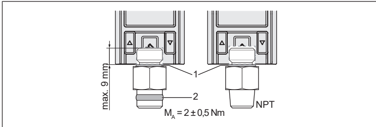
Рис. 17: Двойной ниппель для датчика давления (1 = уплотнительное кольцо, 2 = тефлоновое уплотнительное кольцо)
