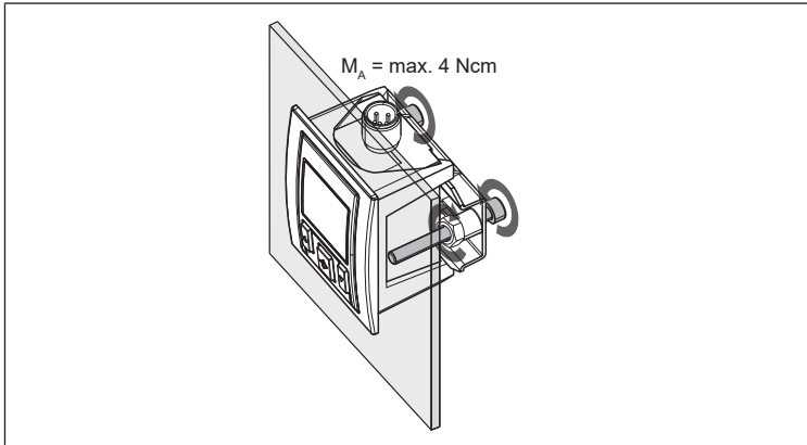
Рис. 16: Зафиксировать с помощью крепежных винтов и законтрить
