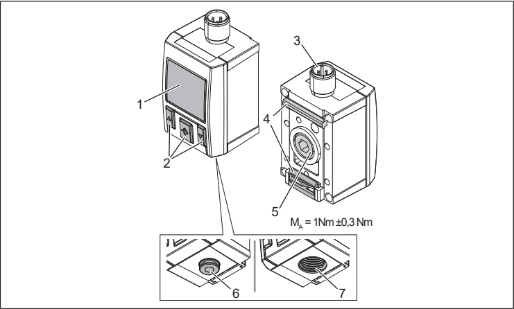
Рис. 1: Обзор устройства
