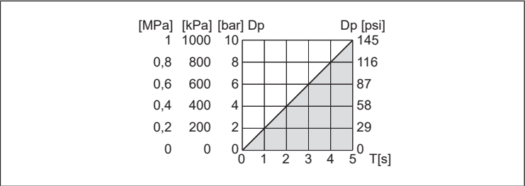
Bild 18: Tillåten periodlängd T (grått område) i förhållande till tryckfluktuationen \Delta p
