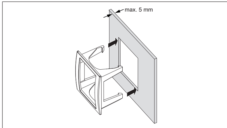
Bild 13: Sätt in frontramen i hålurskärningen
