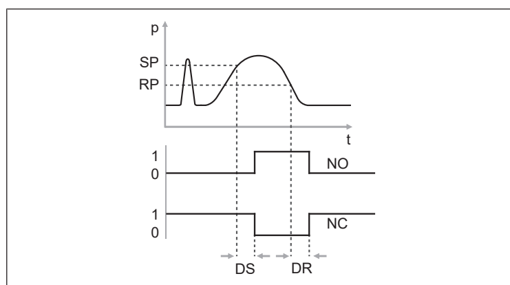
Bild 6: Fördröjningstider
