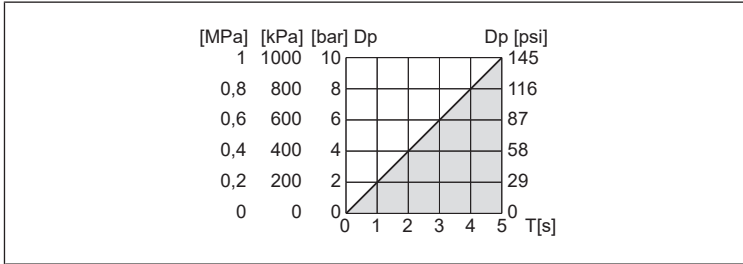
Рис. 18: Допустимая продолжительность периода Т (область серого цвета) в зависимости от колебаний давления Δp
