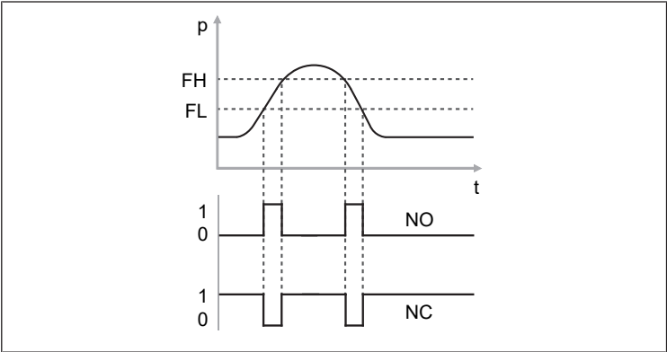
Abb. 5: Fensterfunktion
