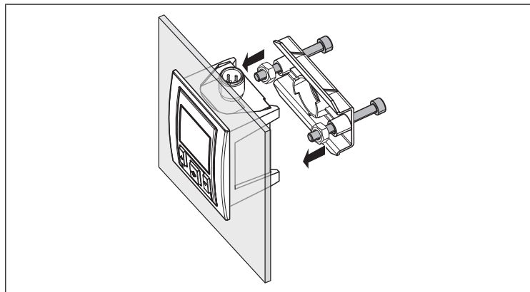
Bild 15: Sätt på monteringssatsen på den nedre fästklämman på tryckvakten och haka i den
