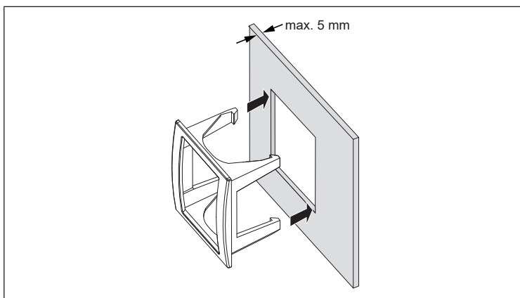
Fig. 13: Insertar el bastidor frontal en el recorte del orificio
