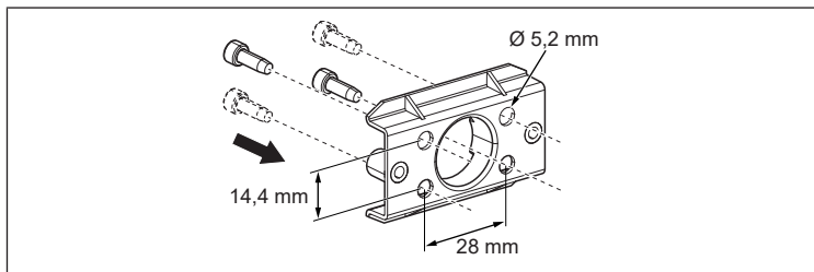
Bild 9: Sätt fast monteringssats R412010405 med 2 skruvar
