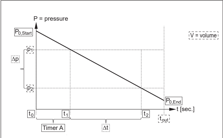
Рис. 23: Кривая утечки
