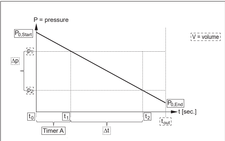
Bild 23: Läckagekaraktäristik
