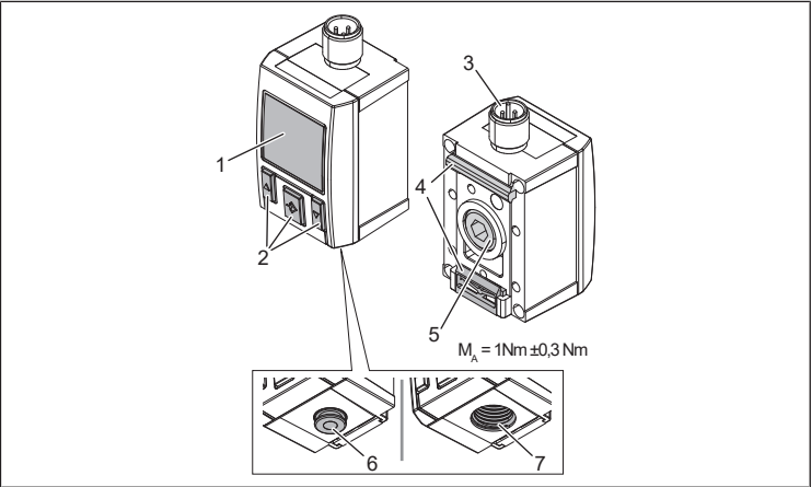
Fig. 1: Panoramica dell'apparecchio
