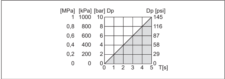
Abb. 18: Zulässige Periodendauer T (grauer Bereich) in Abhängigkeit von der Druckschwankung \Delta p
