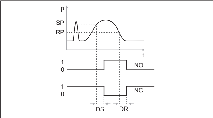
Рис. 6: Время задержки
