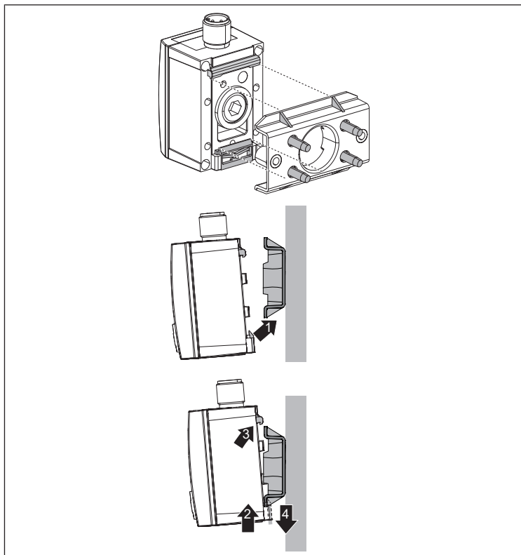
Bild 10: Sätt fast och haka på tryckvakten mitt på monteringssatsen
