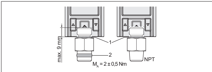
Fig. 17: Manchon double pour capteur de pression (1 = joint torique, 2 = bague d'étanchéité PTFE)
