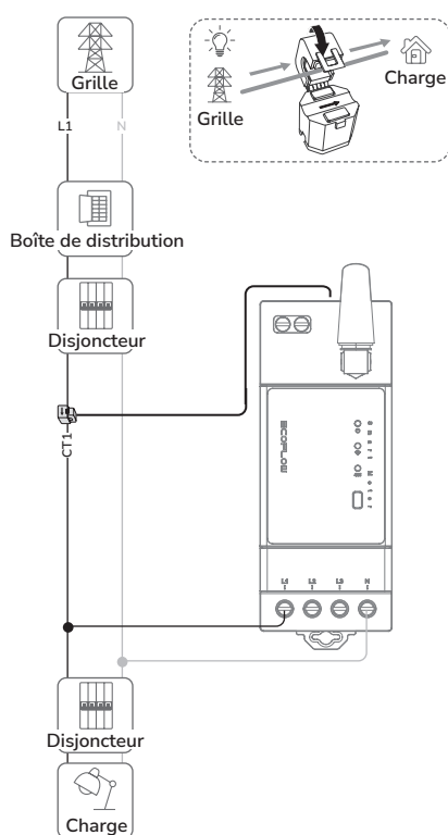
Utilisation comme compteur monophasé
