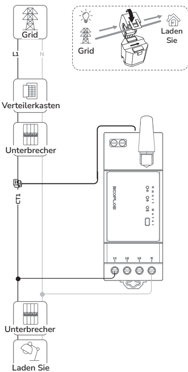
Verwendung als Einphasen-Zähler
