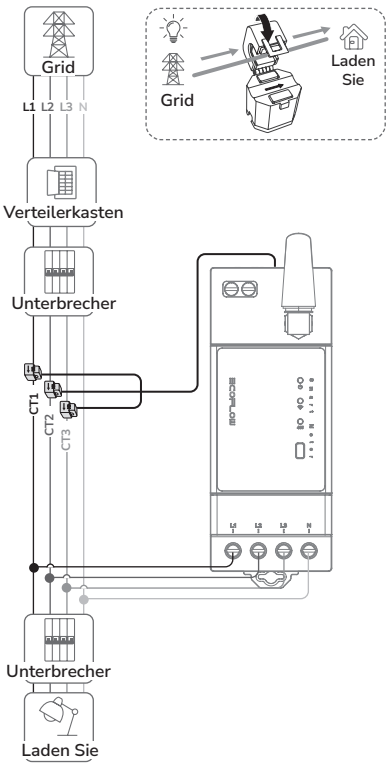
Verwendung als Drehstromzähler
