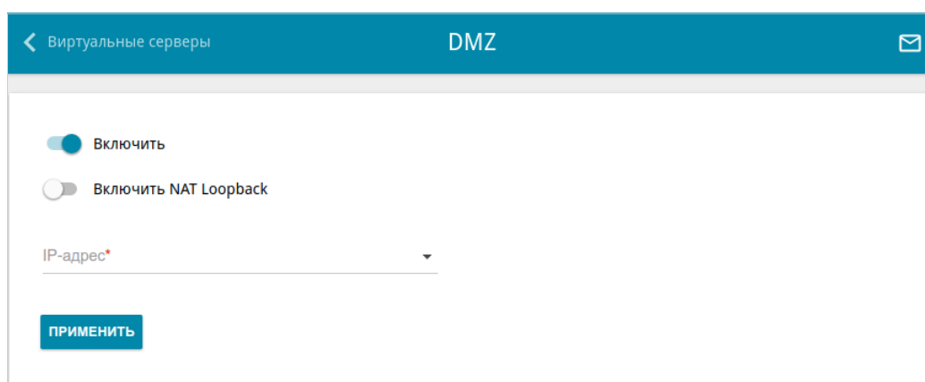
Рисунок 128. Страница Межсетевой экран / DMZ .
