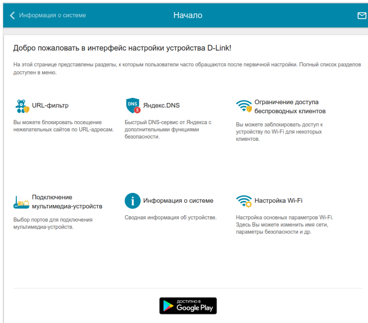
Рисунок 16. Страница Начало .
