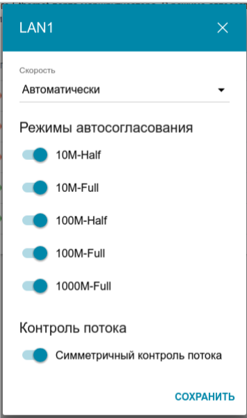
Рисунок 105. Окно изменения настроек порта маршрутизатора.
