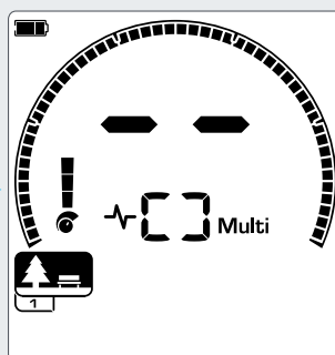
وضع جميع المعادن فعال - تكون جميع نطاقات ميزان التمييز مضبوطة.
