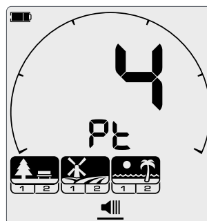
نافذة تعديل وحدة نغمة التمييز - وضع الحديقة والملعب والشاطئ.
