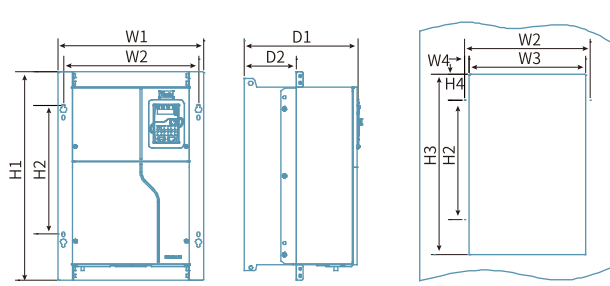
Trifasico CA 380V Diagrama de montaje de 110 ~ 200kW
