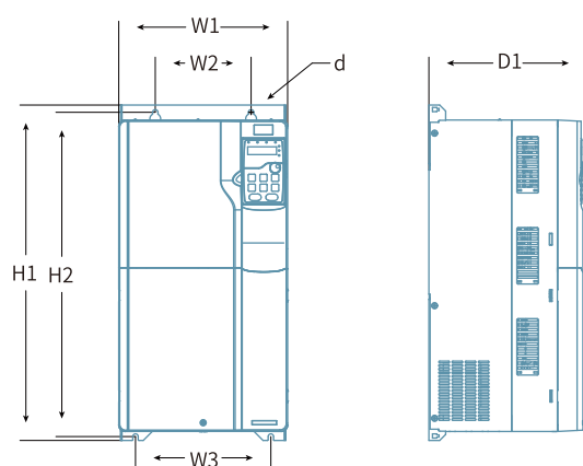
Trifásico CA 380V Diagrama de montaje de 55 ~ 90kW
