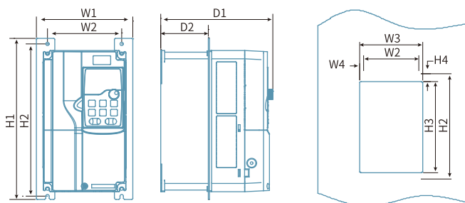
Trifasico CA 380V Diagrama de montaje de 30 ~ 90kW
