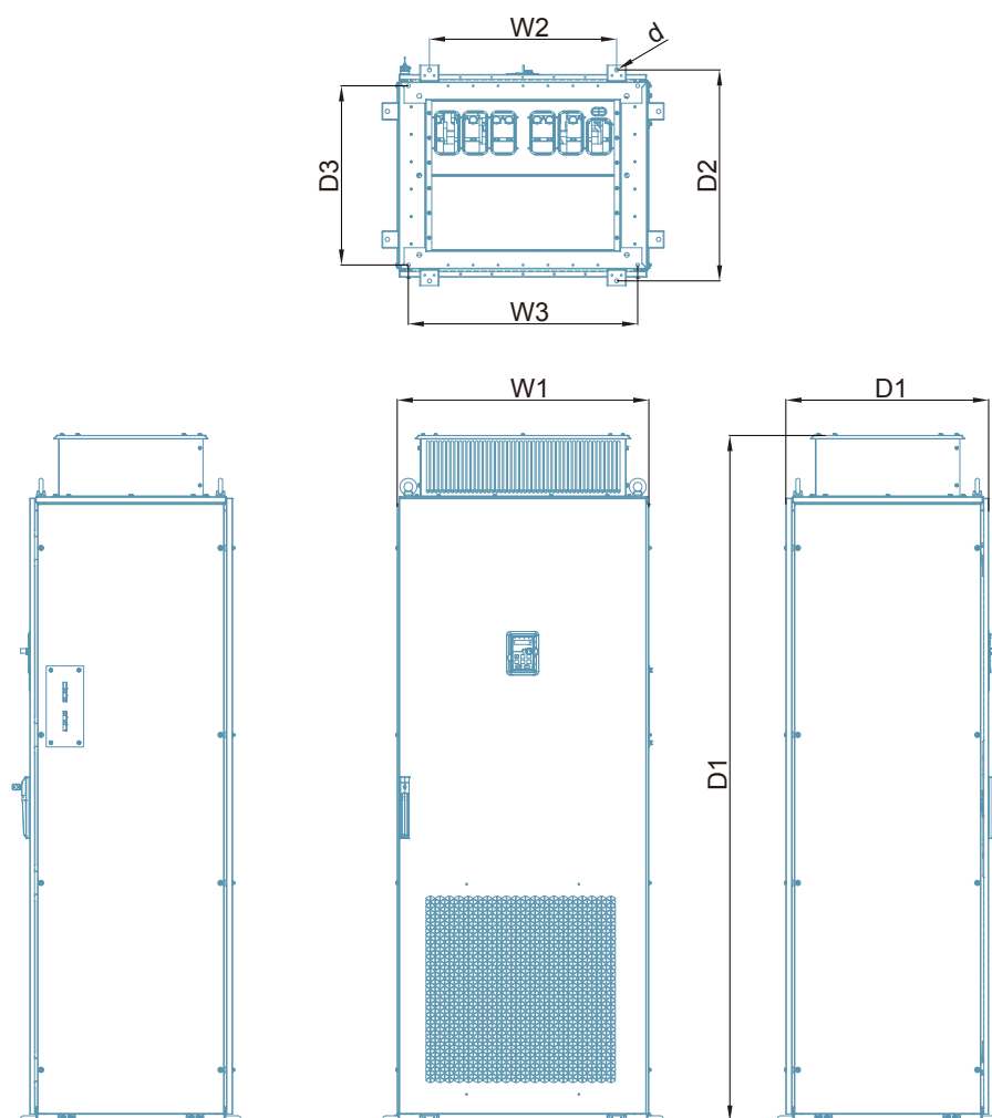
Trifásico CA 380V Diagrama de instalación del modelo 710-800kW
