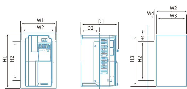
Trifasico CA 380V Diagrama de montaje de 11 ~ 22kW
