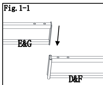
Fig.1-1: Insert long screen1 (D) into long screen 2(E).
