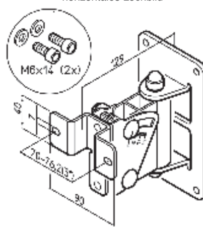
horizontales Lochbild
