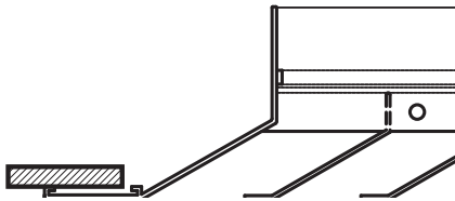
Tegular (-8)
