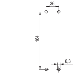
Bohrbild / Drilling pattern / Plan de perçage / esquema de talandros / schema di foratura / esquema de furação / Delik resmi / Расположение отверстий / 钻孔图
