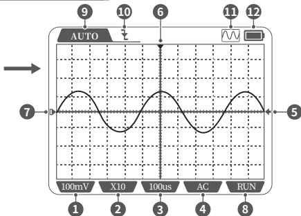
示波器界面
