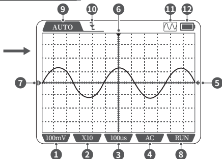
Интерфейс осциллографа
