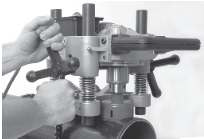
Figura 11 – Perforadora en funcionamiento
