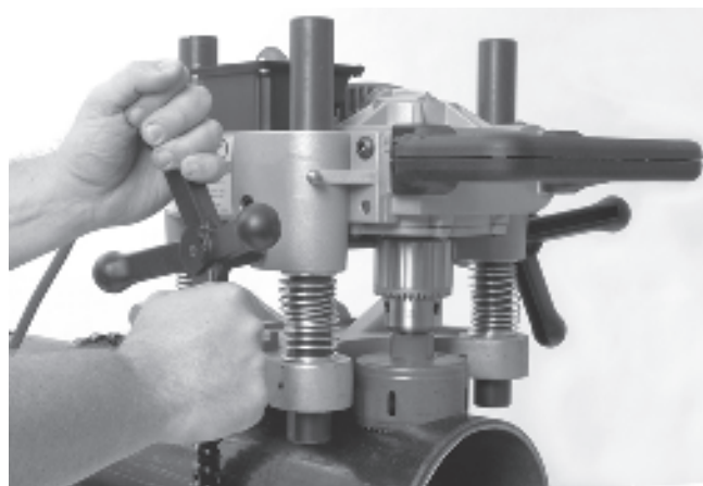
Figure 11 – Utilisation de la scie à cloche
