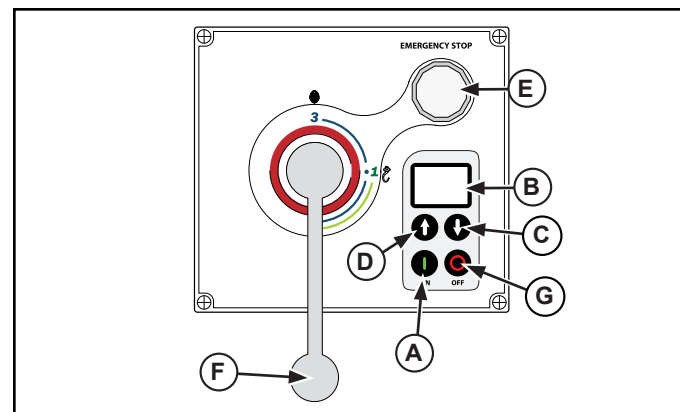
Figure 7. Panneau de commande du mélangeur 40 qt (44 l).
