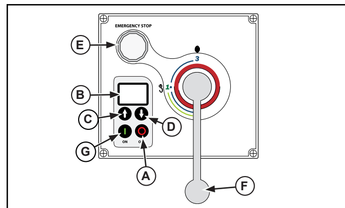
Figure 8. Panneau de commande du mélangeur 60 qt (66 l).
