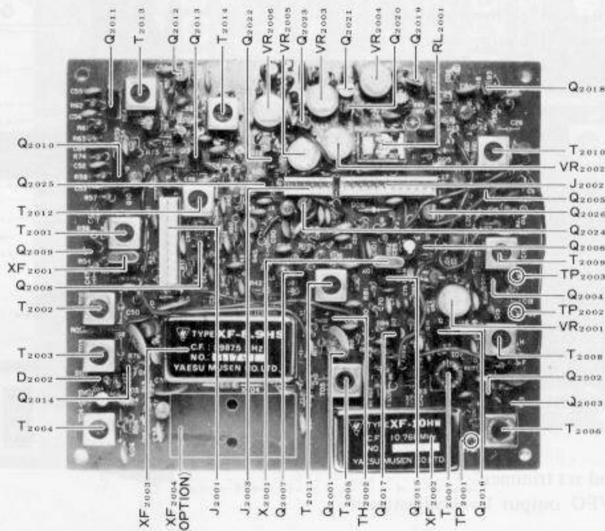
IF UNIT
