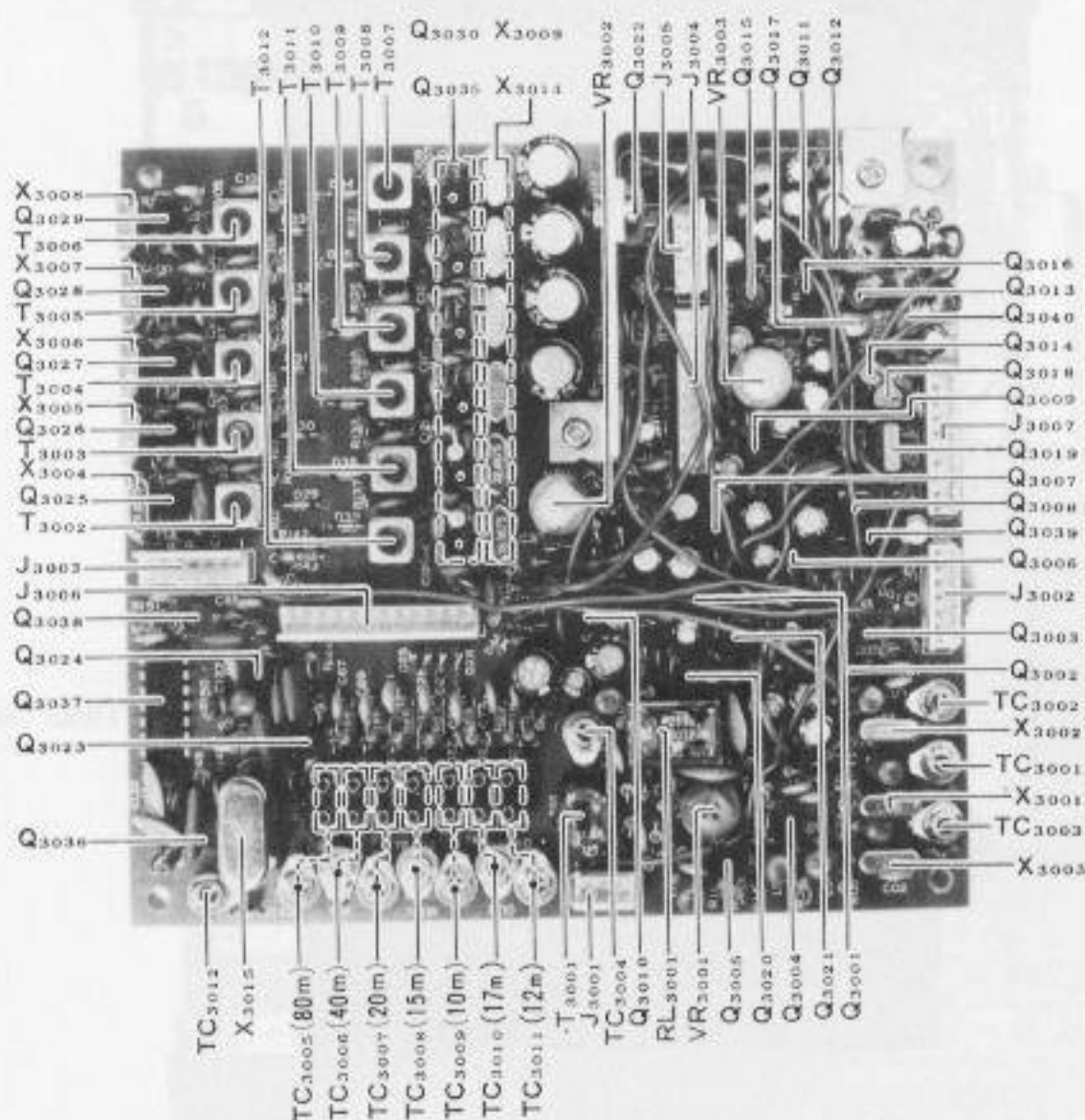
AF UNIT
